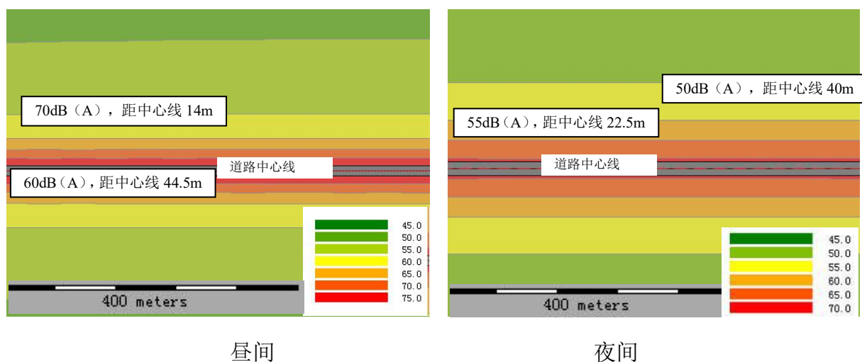
图 12 2026 年富民路西延（濮上路-濮水路）噪声等声级线图
