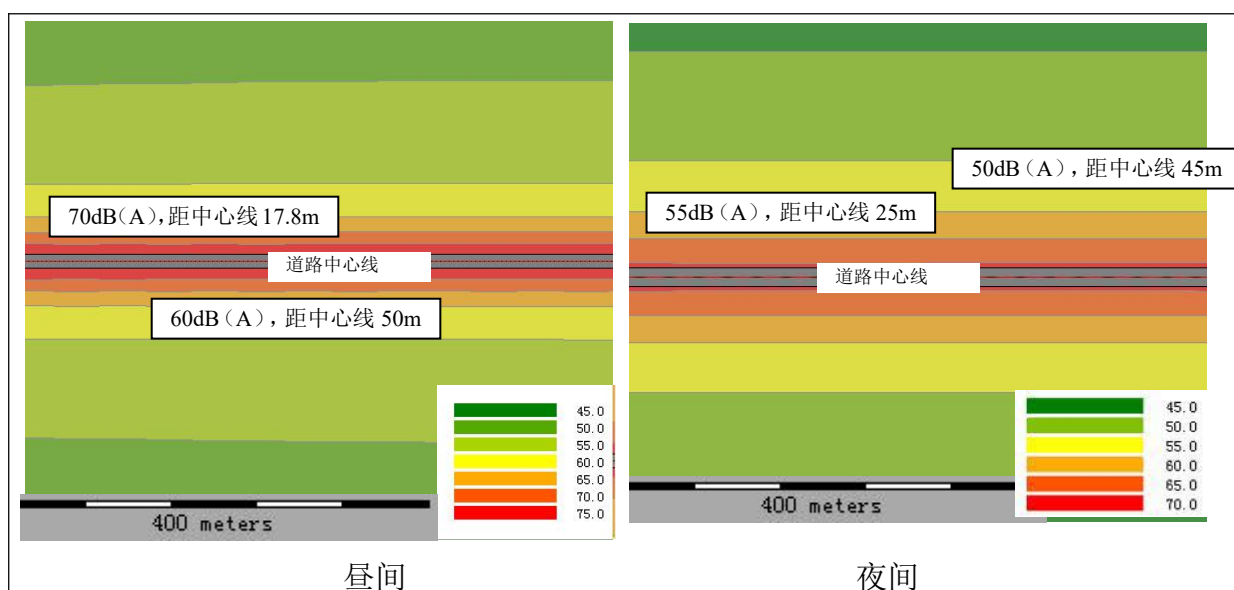
图 13 2035 年富民路西延（濮上路-濮水路）噪声等声级线图
