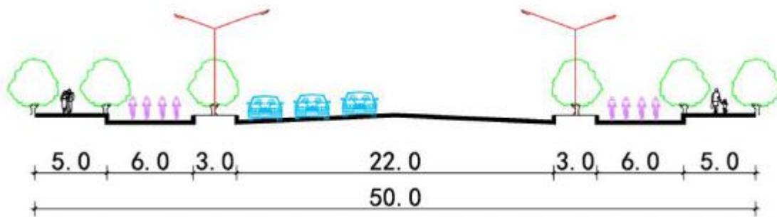
图2 富民路西延（濮上路-濮水路）断面图
