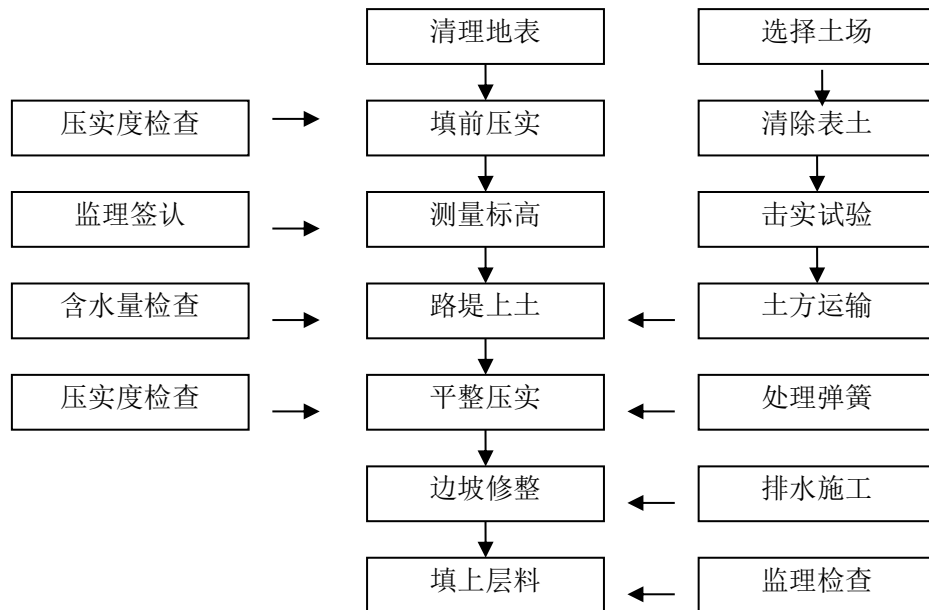
图5 地基填方施工工艺图
