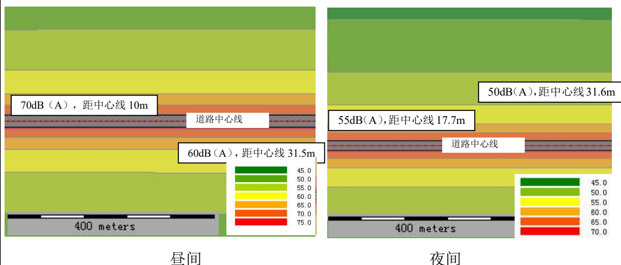
图 11 2021 年富民路西延（濮上路-濮水路）噪声等声级线图
