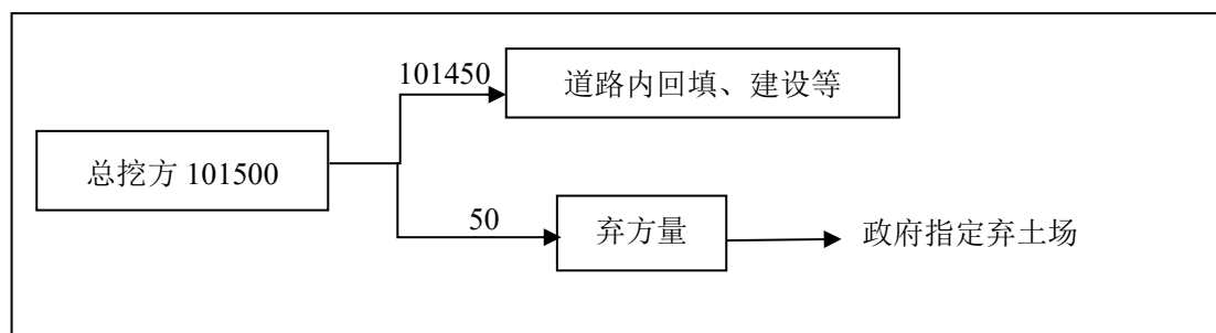
图 3 项目土石方平衡图（单位：m 3 ）
