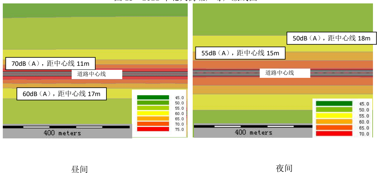
图 16 2026 年北关街噪声等声级线图
