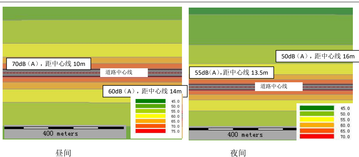
图 15 2021 年北关街噪声等声级线图
