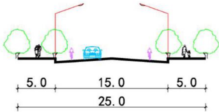
图2 北关街（铁丘路-红旗路）断面图
