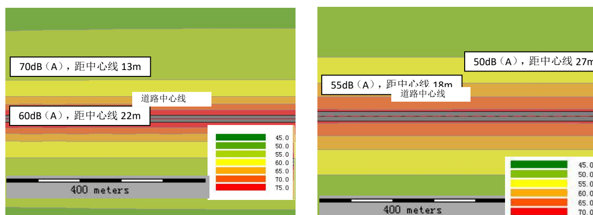
图 12 2026 年吉庆路南延噪声等声级线图
