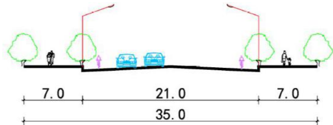
图 2 吉庆路南延（富民路-国庆路）断面图
