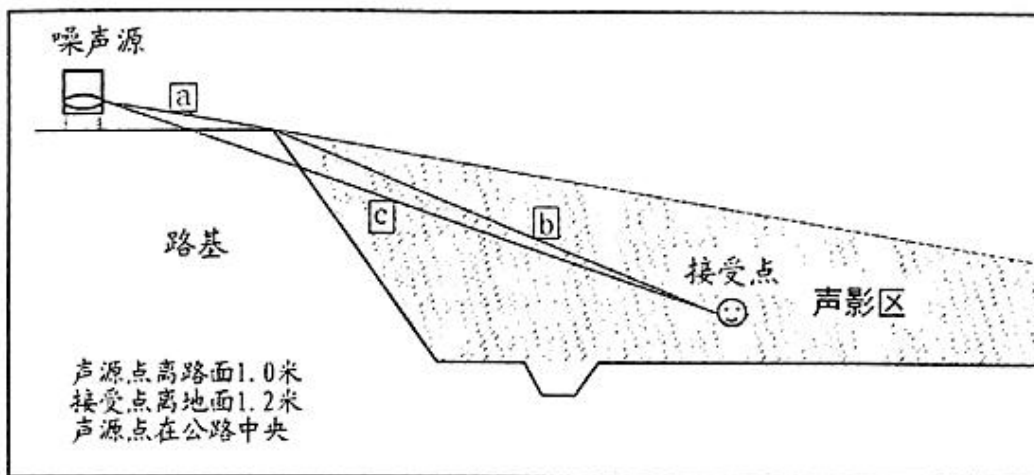
图9 声程差 \delta 计算示意图
