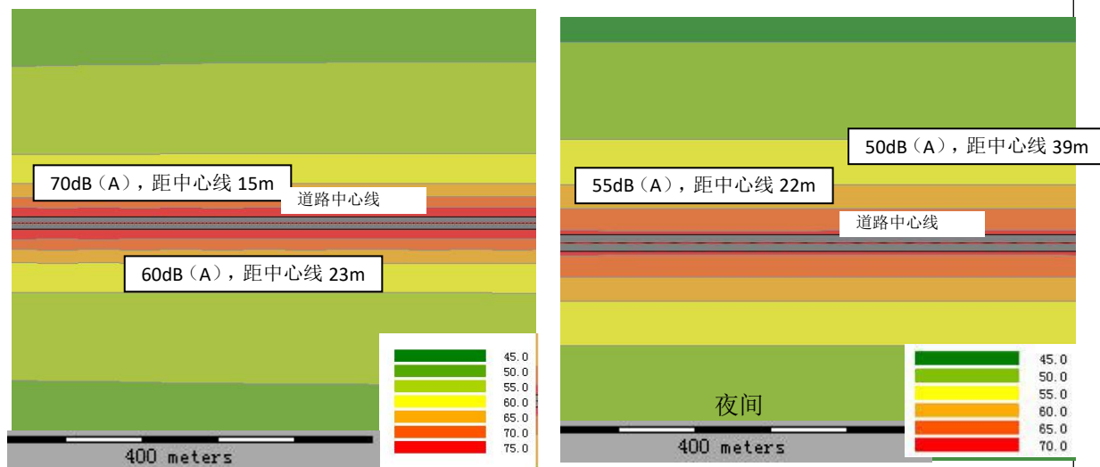
图 13 2035 年吉庆路南延噪声等声级线图
