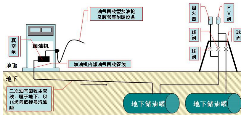
图4 加油油气回收系统基本原理图
