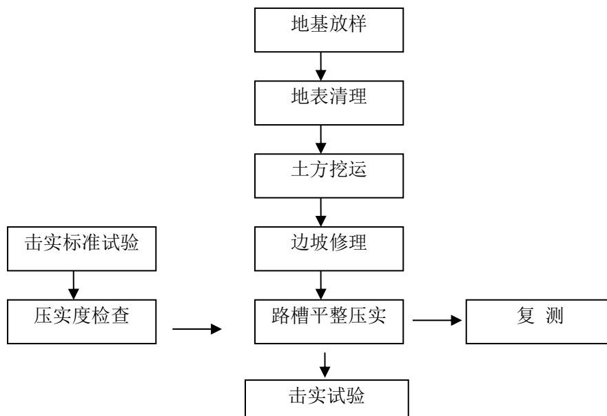
图4 路基挖方施工工艺图
