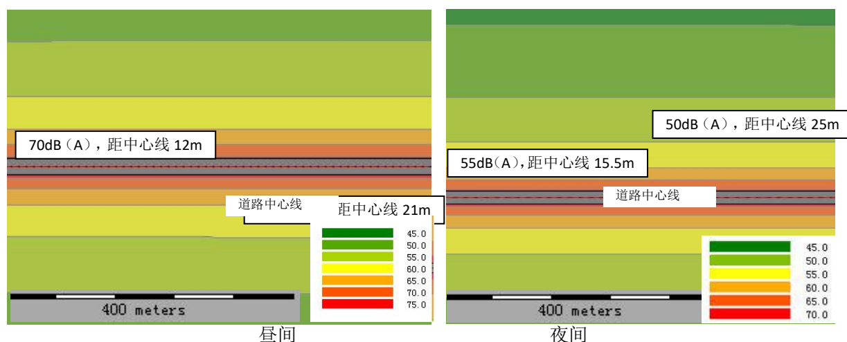
图 11 2021 年富民路（盘锦路-106 国道）噪声等声级线图
