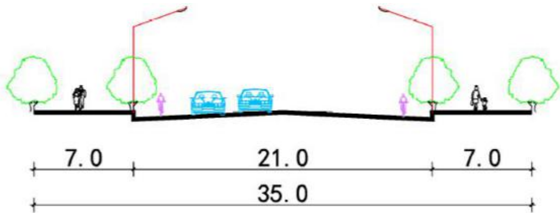
图2 富民路（盘锦路-106 国道）断面图
