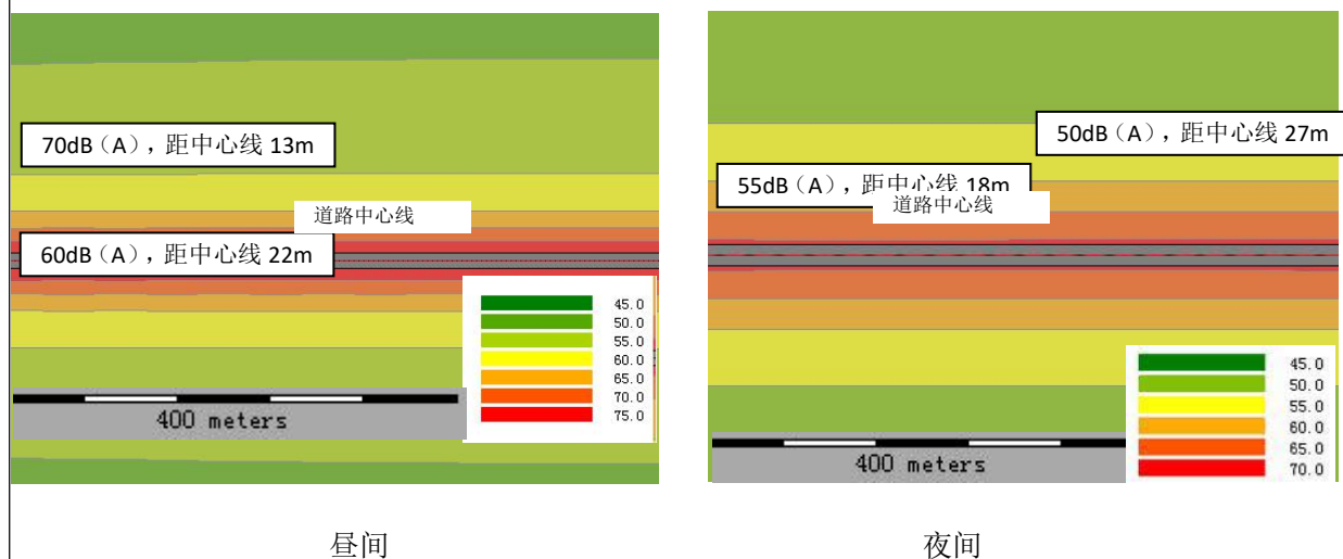
图 12 2026 富民路（盘锦路-106 国道）噪声等声级线图
