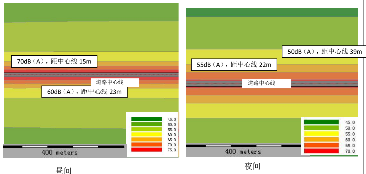
图 13 2035 年富民路（盘锦路-106 国道）噪声等声级线图
