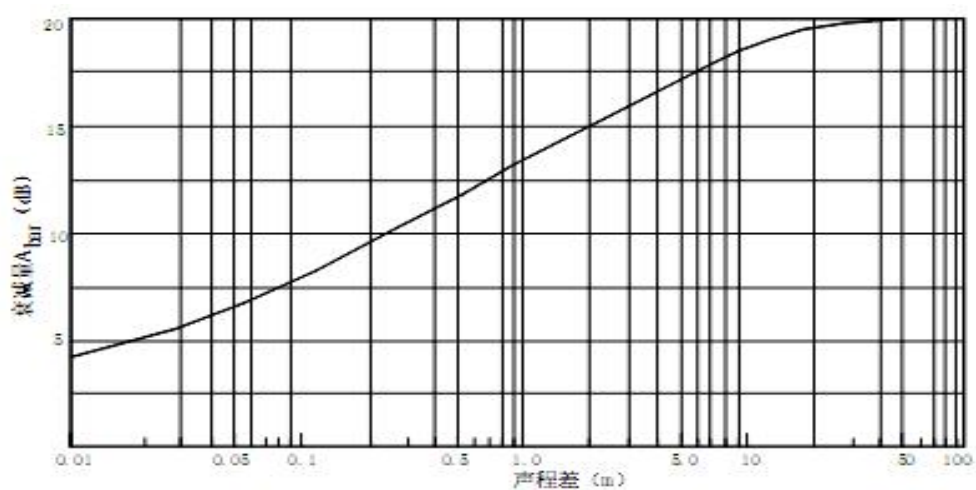
图10 噪声衰减量 A_{\bar{a}} 与声程差 \delta 关系曲线
