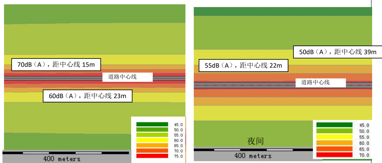
图 17 2035 年富民路中段噪声等声级线图
