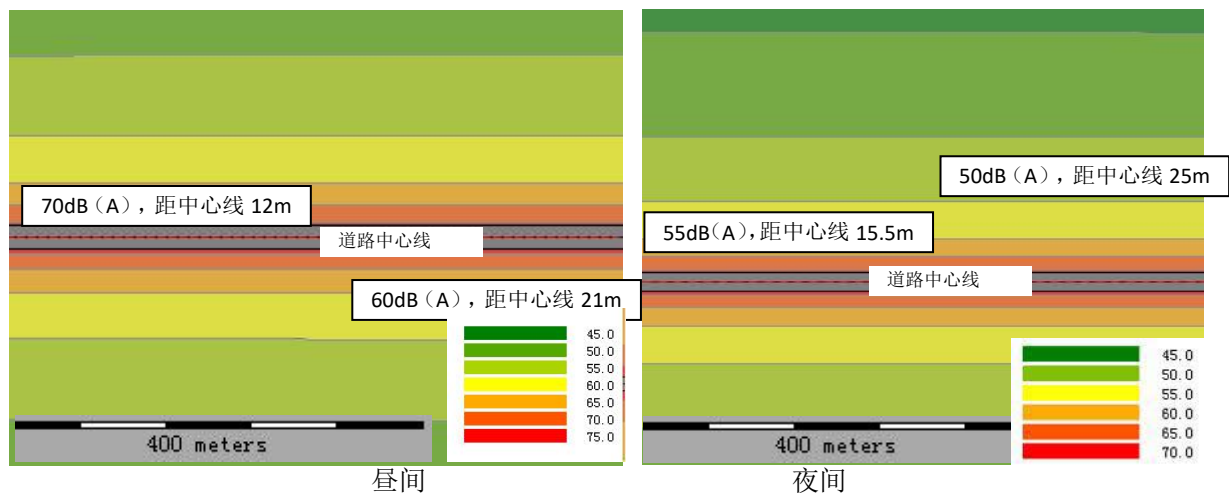
图 15 2021 年富民路中段噪声等声级线图
