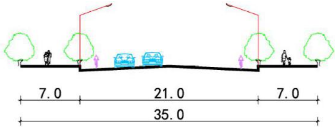
图 2 富民路（濮上路-云峰路）断面图
