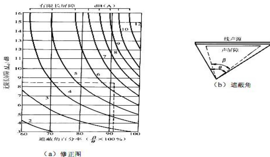
图9 有效长度的声屏障及线声源的修正图
