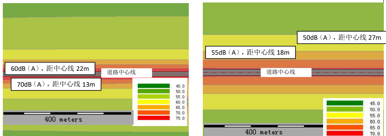
图 16 2026 年富民路中段噪声等声级线图
