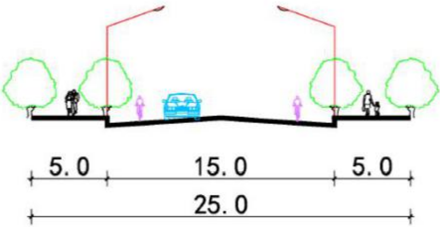
图 2 御井街（红旗路-富民路、龙苑路-站南路）断面图
