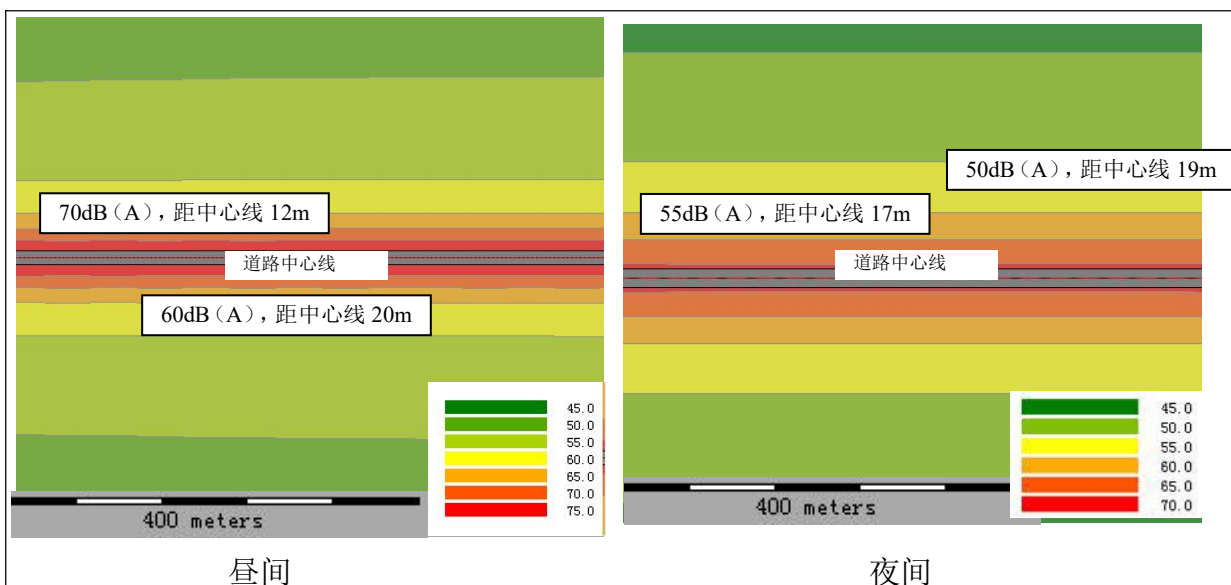
图 17 2036 年御井街噪声等声级线图
