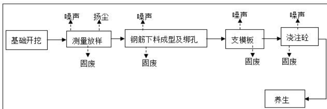
图9 系梁、承台施工流程示意图
