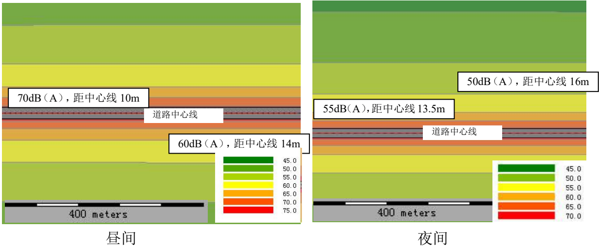
图 15 2022 年御井街噪声等声级线图
