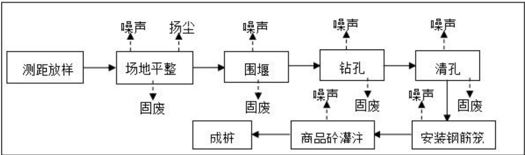
图 8 钻孔灌注桩柱施工流程示意图
