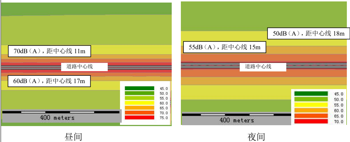
图 16 2027 年御井街噪声等声级线图
