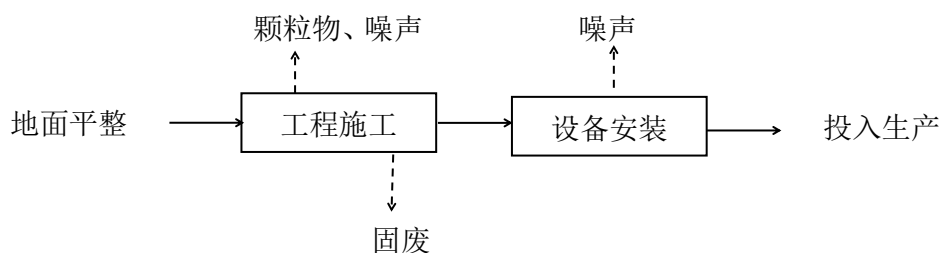
图 1 施工期工艺流程及产物环节图
