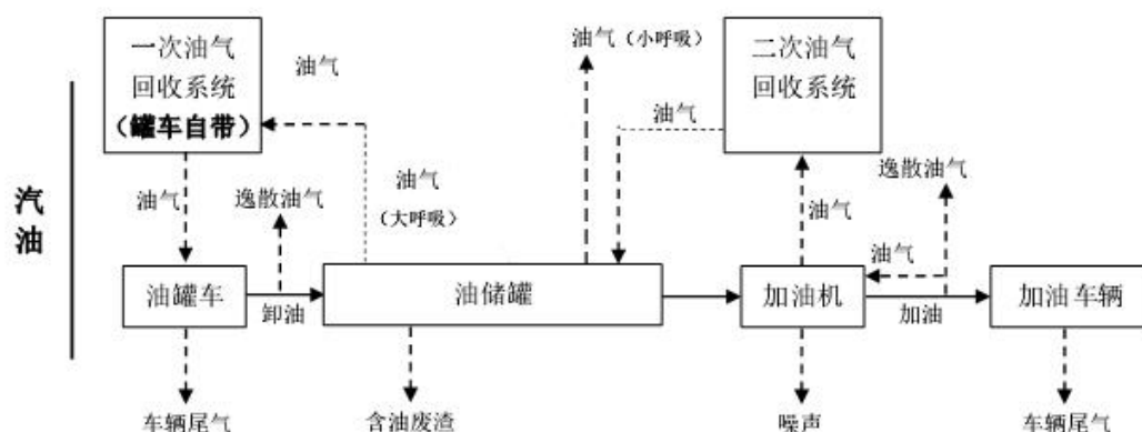
图 2 项目运营期工艺流程及产污环节示意图
