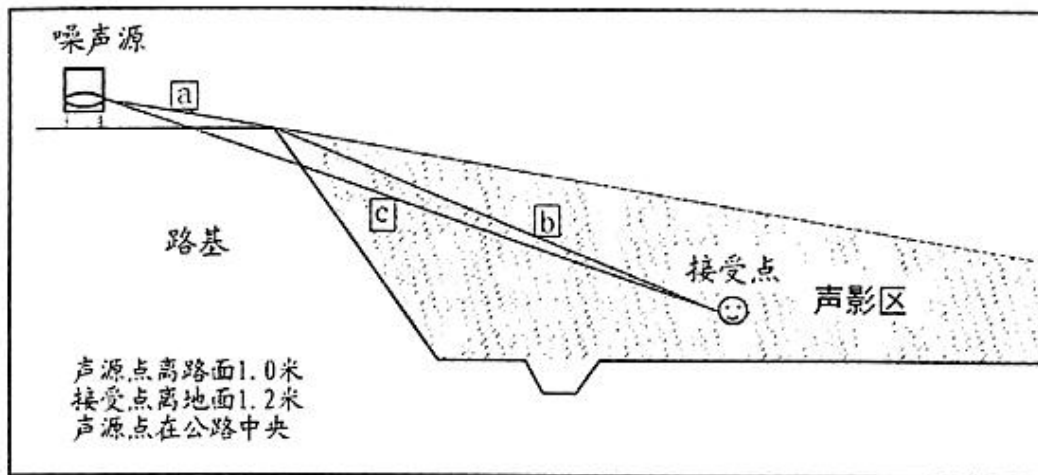
图 12 声程差 \delta 计算示意图
