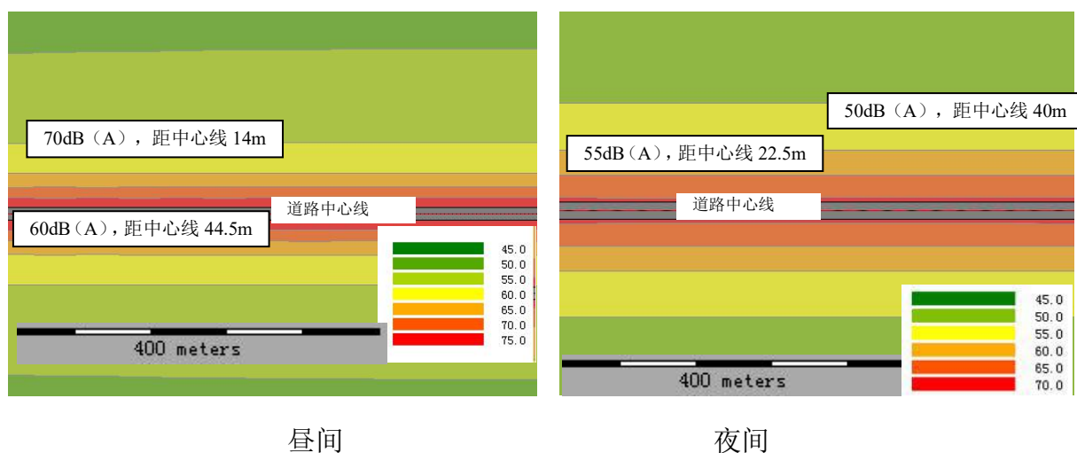
图 15 2026 年新东路噪声噪声等声级线图
