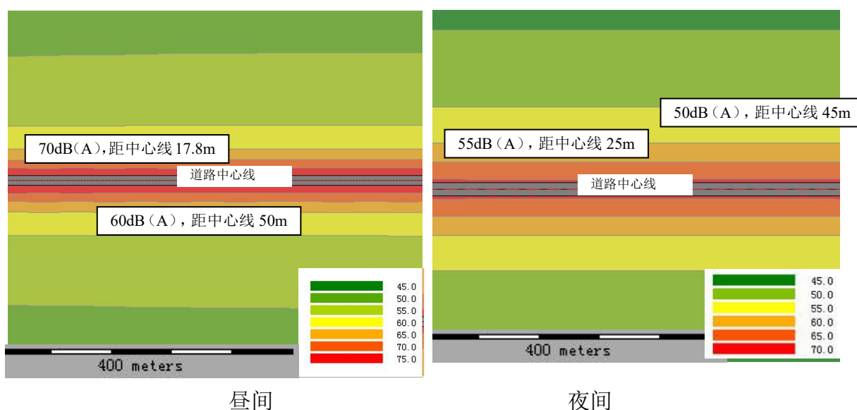
图 16 2035 年新东路噪声噪声等声级线图
