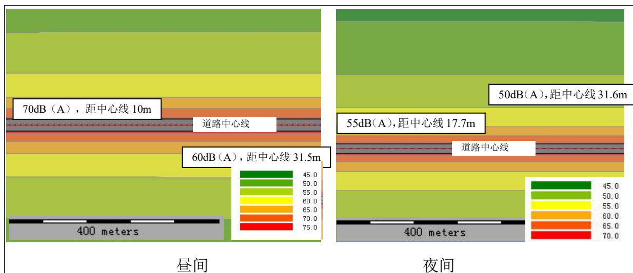
图 14 2021 年新东路噪声等声级线图
