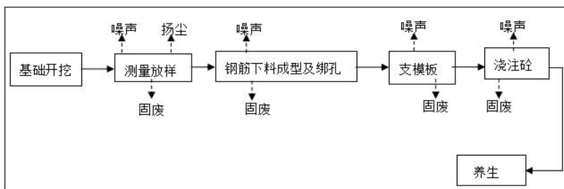
图 8 系梁、承台施工流程示意图
