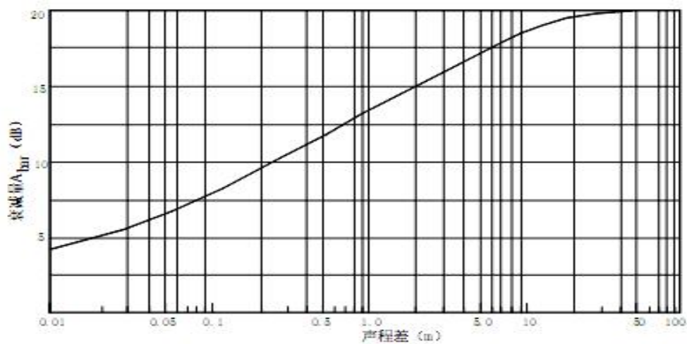
图 13 噪声衰减量 A_{bar} 与声程差 \delta 关系曲线
