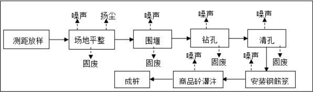
图 7 钻孔灌注桩柱施工流程示意图
