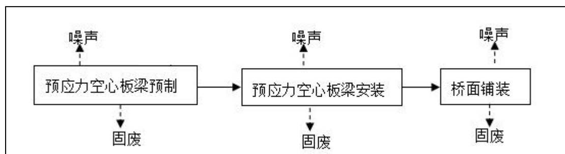
图 9 桥梁上部结构施工流程示意图
