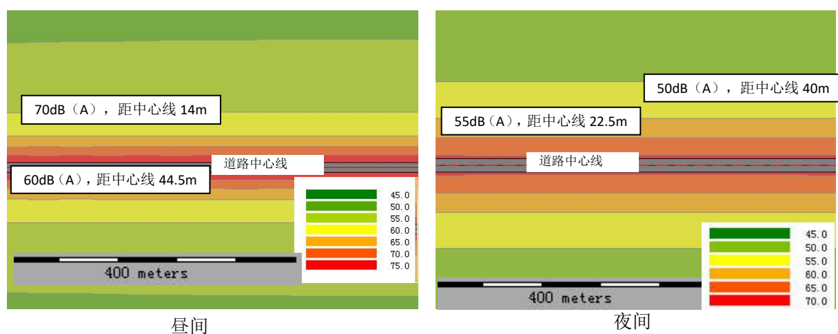
图 11 2026 年红旗路东延噪声噪声等声级线图
