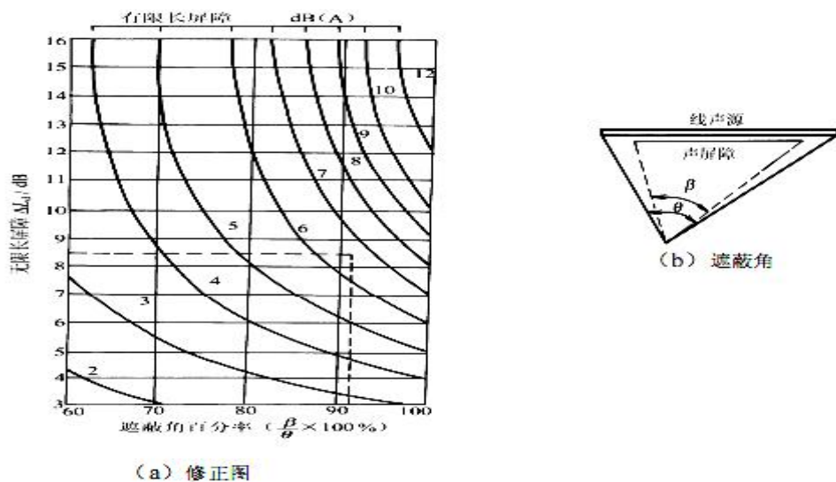
图7 有效长度的声屏障及线声源的修正图
