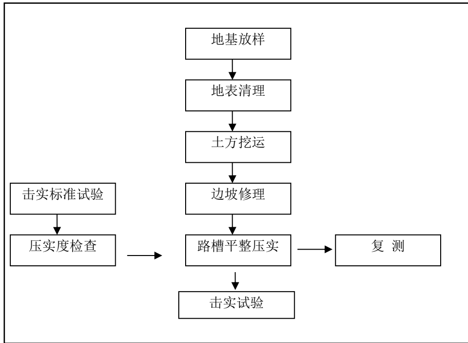
图3 路基挖方施工工艺图
