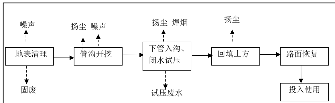
图5 管线铺设流程示意图
