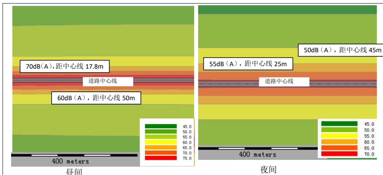
图 12 2035 年红旗路东延噪声等声级线图
