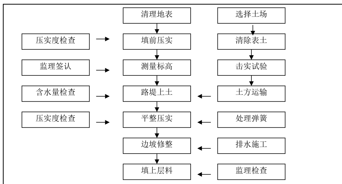
图4 地基填方施工工艺图
