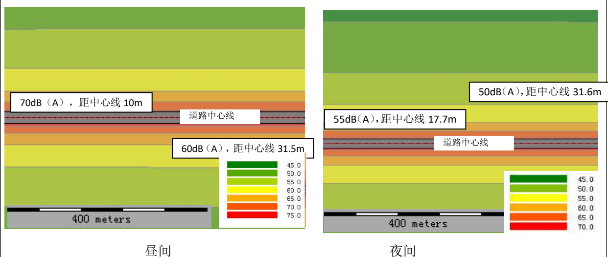
图 10 2021 年红旗路东延噪声等声级线图
