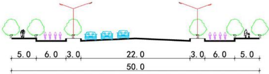
图 2 红旗路东延（盘锦路-106 国道）断面图
