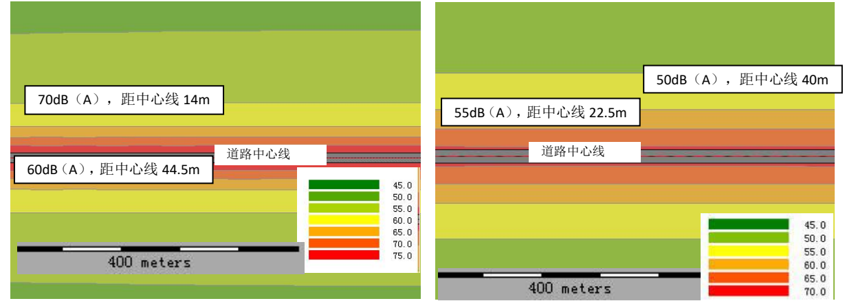
昼间 图 15 2026 年胜利东路噪声等声级线图
