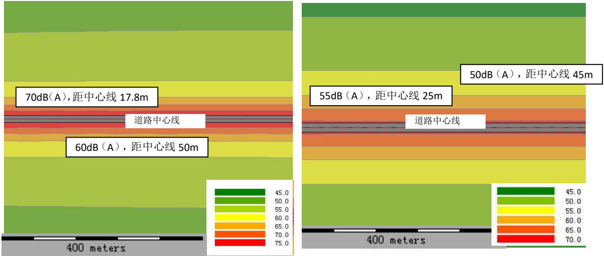
昼间 图 16 2035 年胜利东路噪声等声级线图
