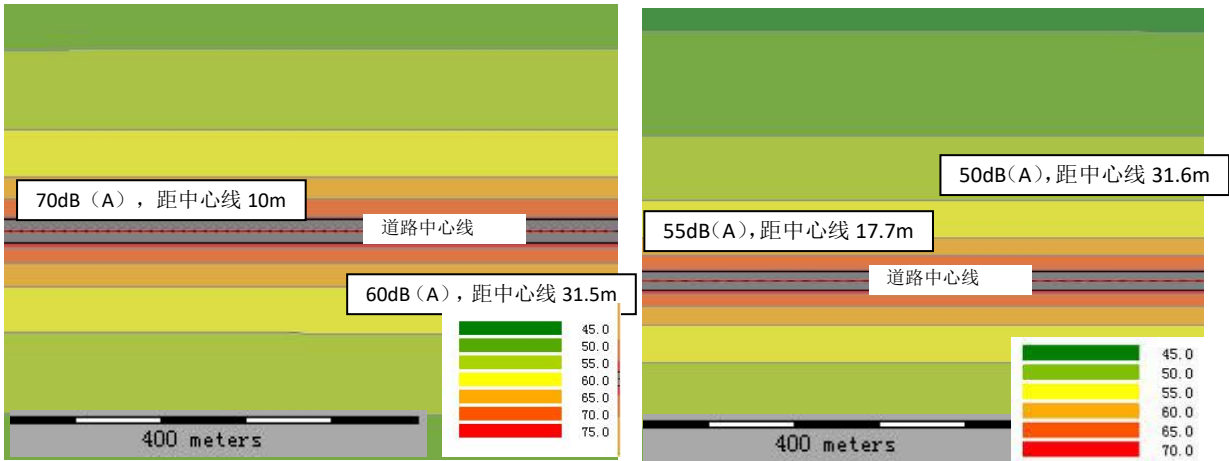
昼间 图 14 2021 年胜利东路噪声等声级线图
