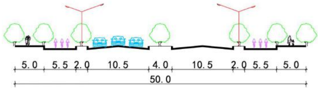
图 2 胜利路（106 国道-龙乡路）断面图
