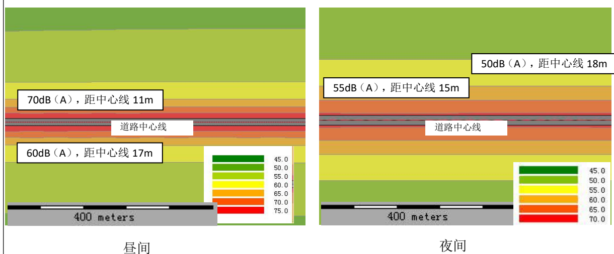
图 15 2026 年花园路噪声等声级线图
