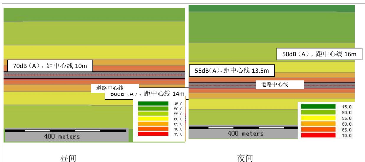
图 14 2021 年花园路噪声等声级线图
