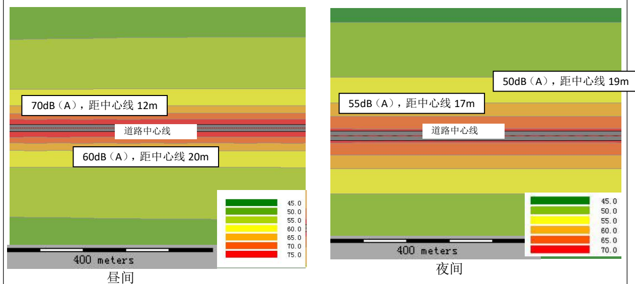
图 16 2035 年花园路噪声等声级线图
