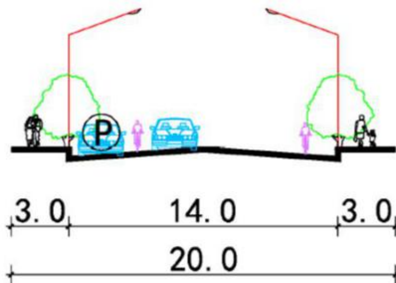
图 2 花园路（文明路-盘锦路）断面图
