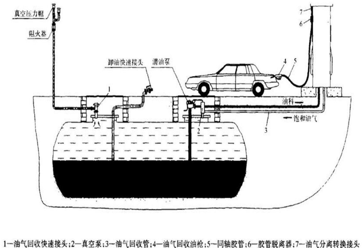
图 4 加油环节油气回收示意图
