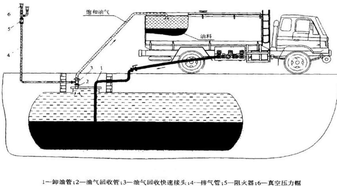
图 3 一级油气回收系统
