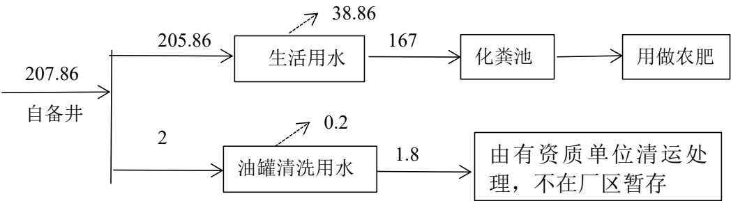
图 5 项目水量平衡图 (m³/a)
