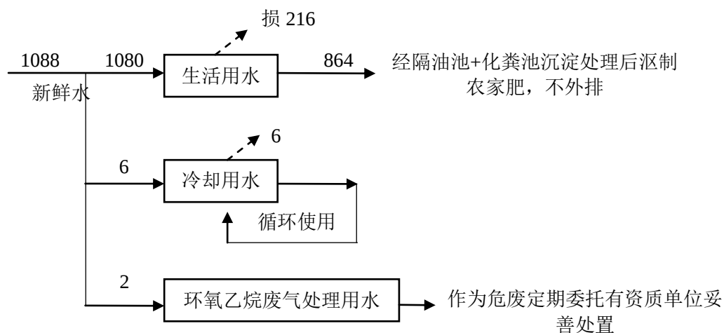
图 5 改扩建项目水平衡示意图 单位：m 3 /a
