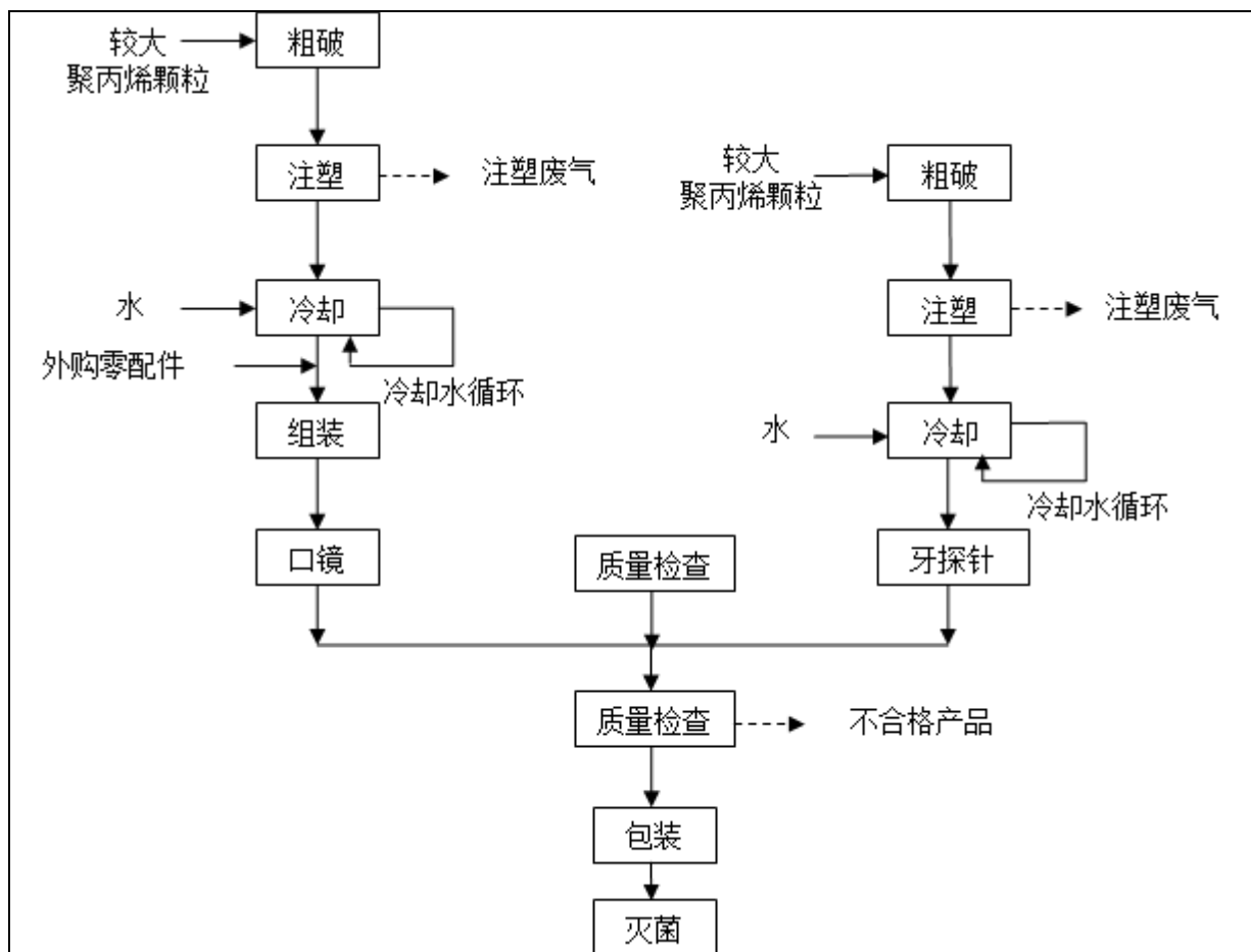
图 2 原有项目生产工艺及产污环节示意图
