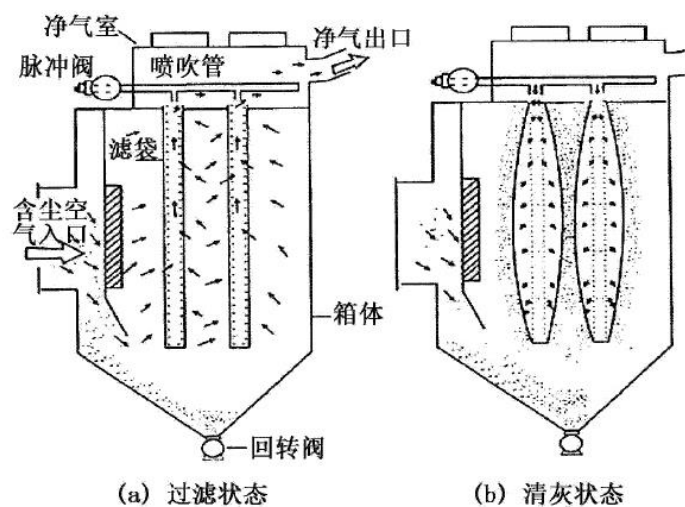
图 4 脉冲袋式除尘器工作示意图
