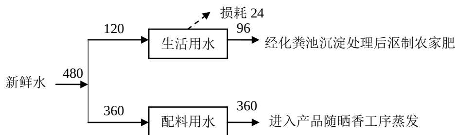
图 3 项目水平衡示意图 单位： \text{m}^3/\text{a}
