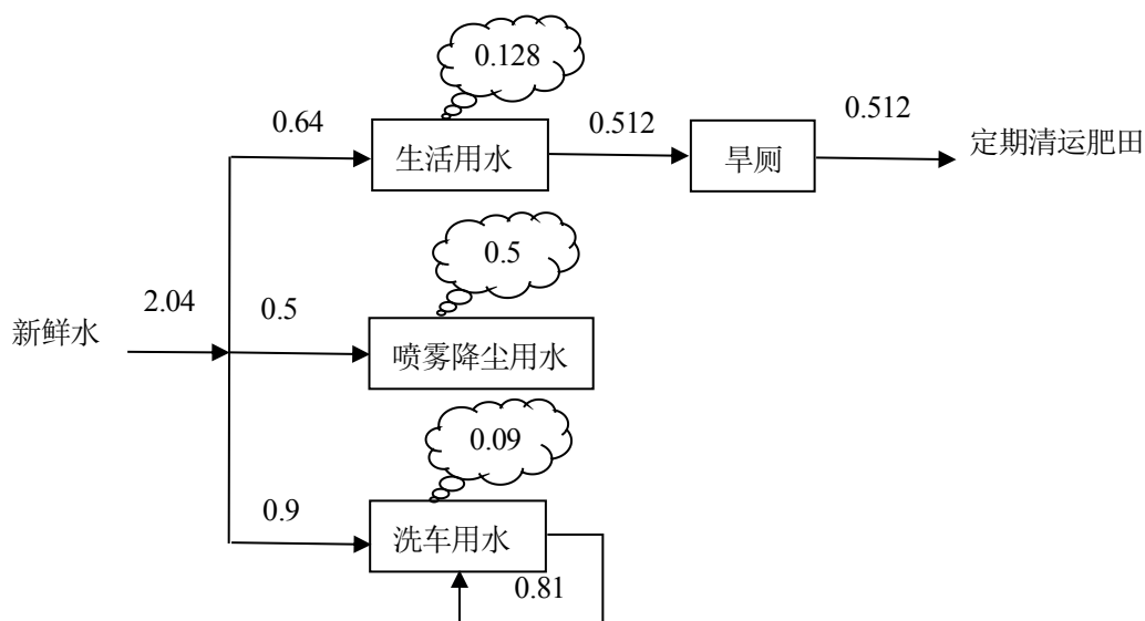
图 1 项目水平衡示意图 单位: \text{m}^3/\text{d}
