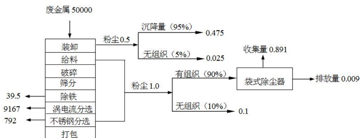
图 4 项目物料平衡图 (单位: t/a)
