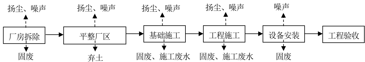
图2 施工期工艺流程及产污节点示意图
