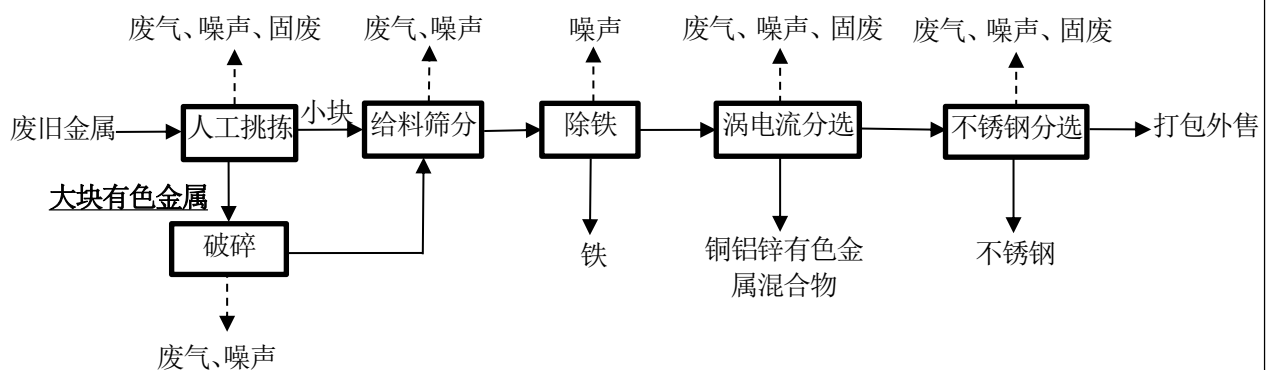
图3 项目运营期工艺流程及产污环节示意图
