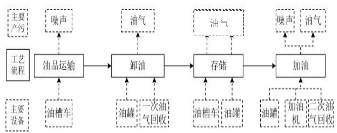
图 1 运营期卸油、加油工艺流程及产污位置框图
