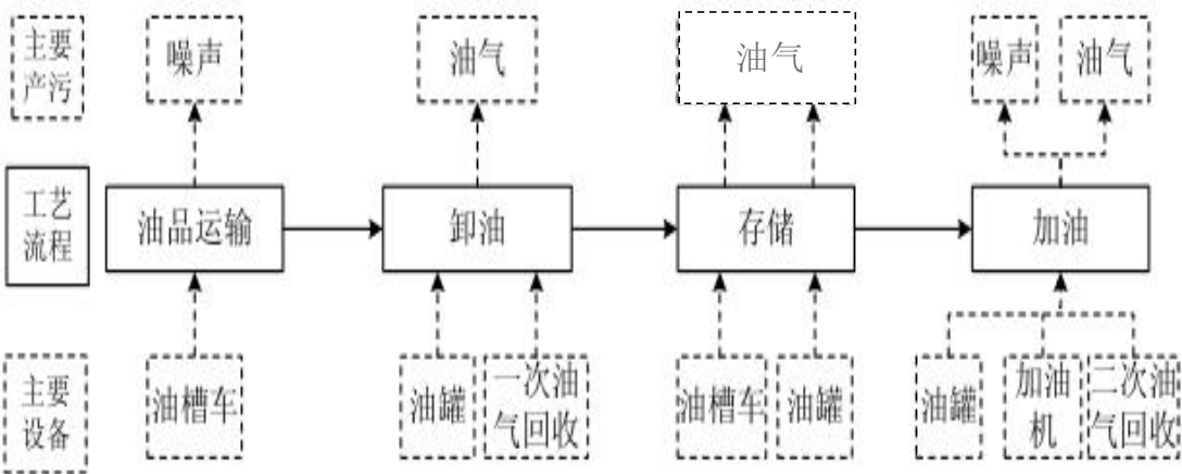
图2 运营期卸油、加油工艺流程及产污位置框图
