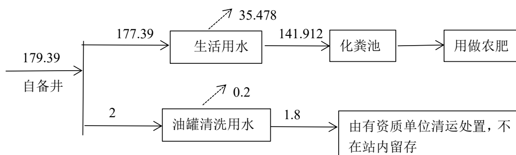
图5 项目水量平衡图 (m 3 /a)
