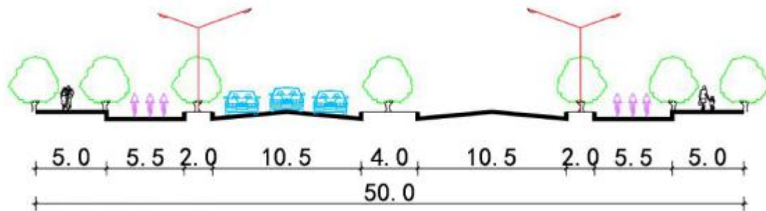
图 2 干城路（工业大道-建设路）断面图
