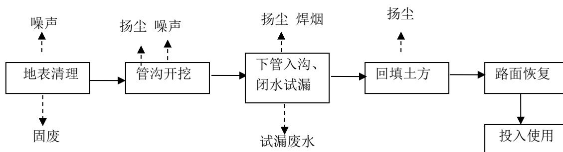
图 7 管线铺设流程示意图
