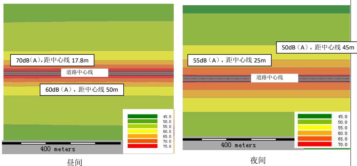
图 18 2036 年干城路噪声等声级线图
