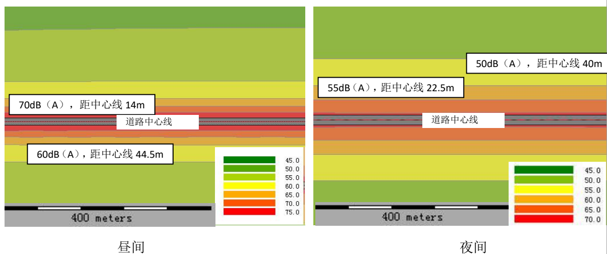
图 17 2026 年干城路噪声等声级线图
