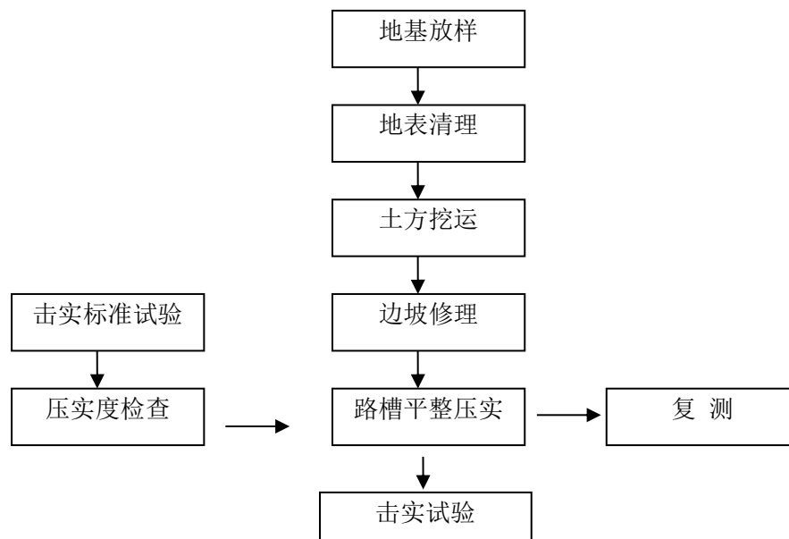
图5 路基挖方施工工艺图
