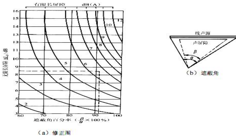
图 12 有效长度的声屏障及线声源的修正图
