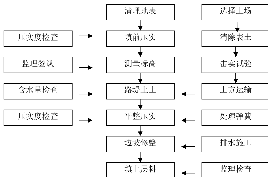
图 6 地基填方施工工艺图
