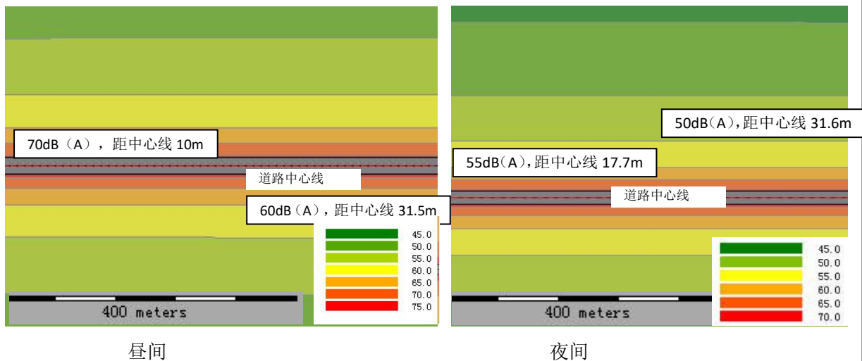
图 16 2021 年干城路噪声等声级线图
